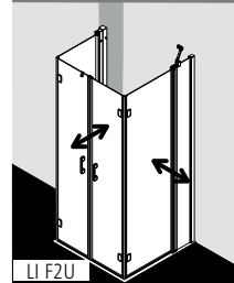
U-Form mit Festfeld: LI F2U als Maßanfertigung siehe Skizze 2
