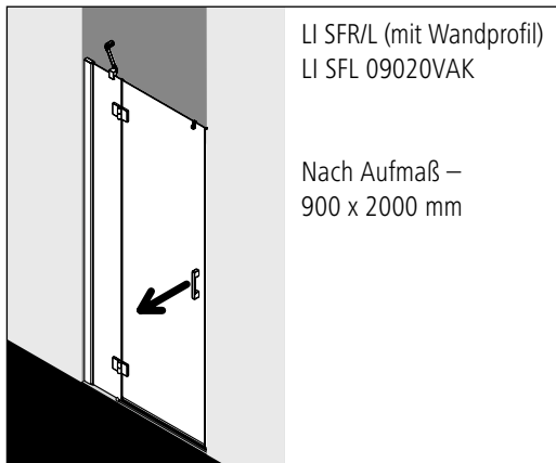
Schwingtür 900 x 2000 mm, Profile silber hochglanz, ESG klar, Preis o. MwSt.
